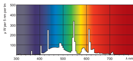
Lichtfarbe TL-D de Luxe /965
