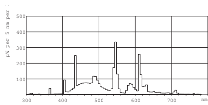
Lichtfarbe TL-D de Luxe /965
